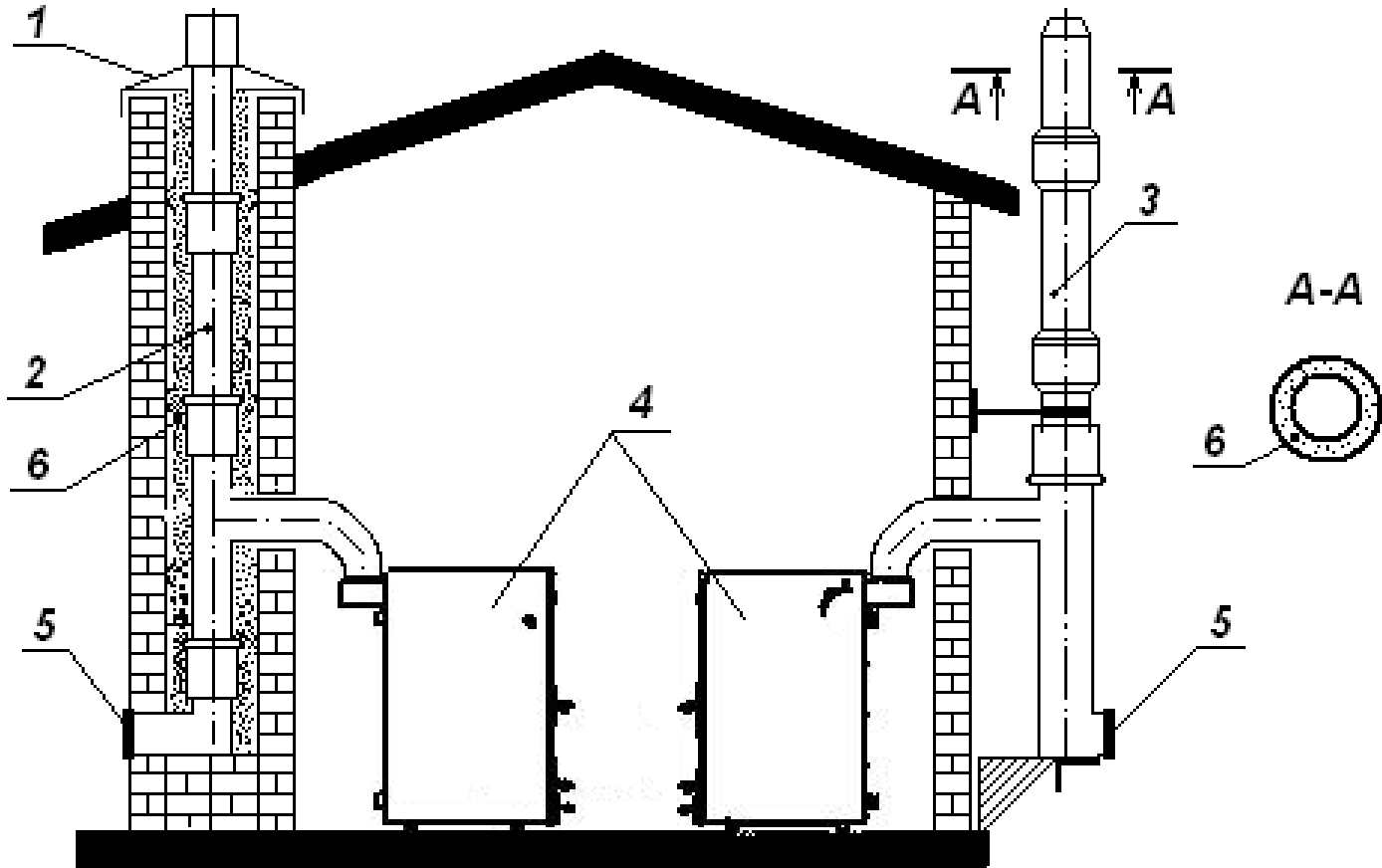
Рисунок 3. Варіанти конструкції димоходу
