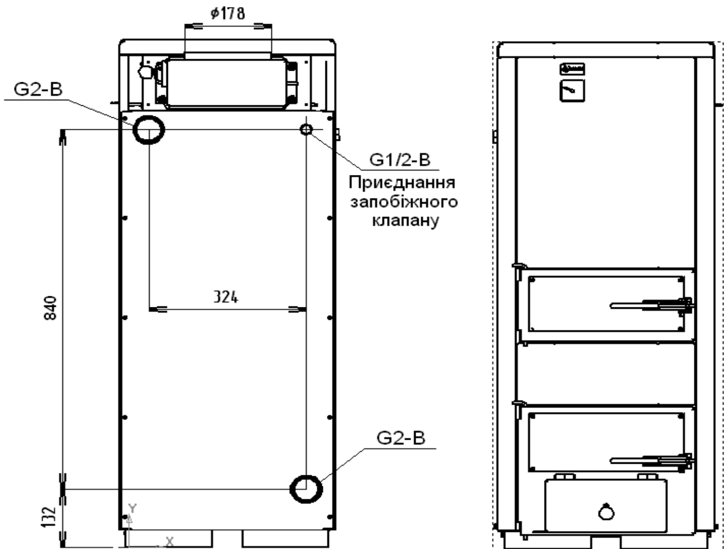
Рисунок 2. Приєднувальні розміри
