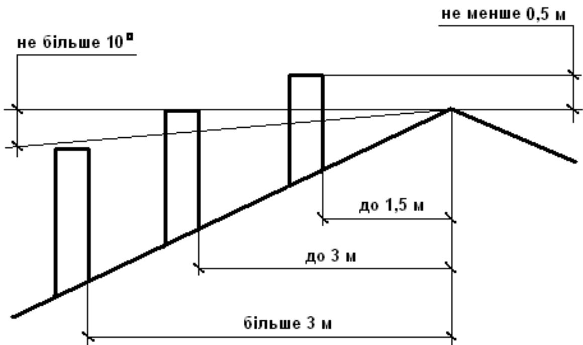
Рисунок 4. Розміщення димоходу
