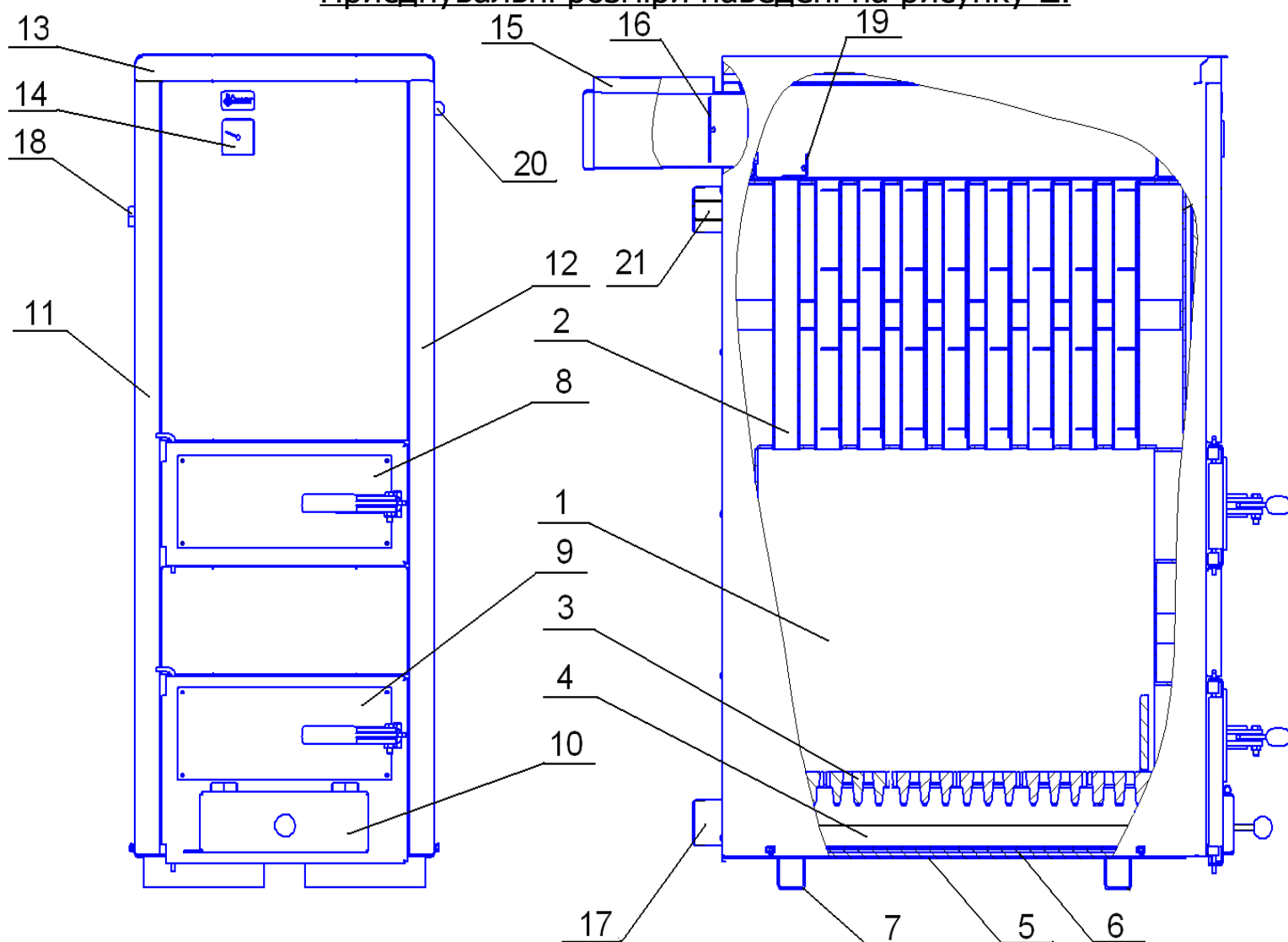
Рисунок 1. Котел опалювальний
